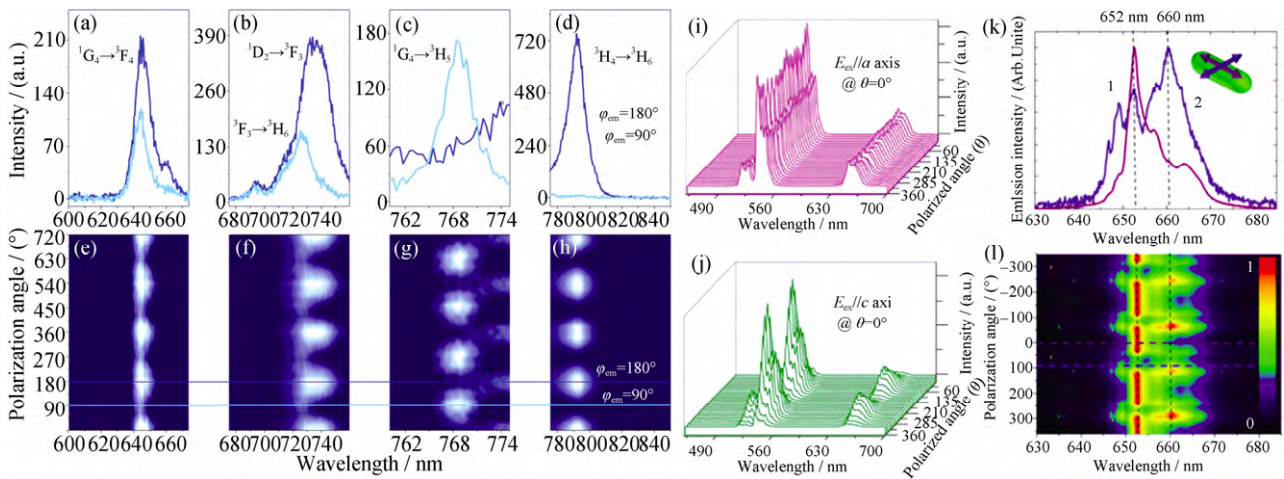
图 5 (a~d)单根 \beta -NaYF 4 : Tm 3+ -Yb 3+ 微米棒的上转换发射光谱图, 分别对应 Tm 3+ 跃迁: (a) 1 G 4 → 3 F 4 , (b) 3 F 3 → 3 H 6 , 1 D 2 → 3 F 3 , (c) 1 G 4 → 3 H 5 , (d) 3 H 4 → 3 H 6 ; (e~h)各跃迁荧光强度随发射偏振角的变化关系; (i, j)单个纳米盘其晶体学 a 轴(i)或 c 轴(j)平行水平面时, 上转换发射光谱随激发偏振角变化; (k)单根 NaYF 4 : Er 3+ , Yb 3+ 纳米棒其处于两个相垂直发射偏振角度时的发射光谱图。曲线 1 和曲线 2 表示发射偏振角平行和垂直纳米棒光轴。插图表示电场下两个不同偏振方向, 产生截然不同的光谱; (l)二维图谱表示红光波段的发射强度随发射偏振角的变化关系 [27,31]
