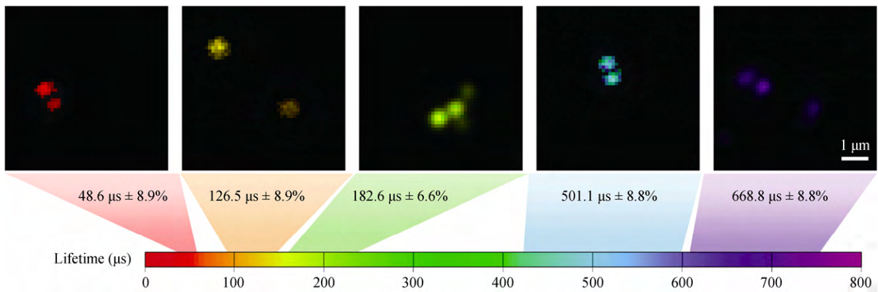
图 6 荧光寿命调节示范, 即 NaYF 4 : Yb, Tm 上转换纳米颗粒的时间分辨共聚焦图像 [10]
