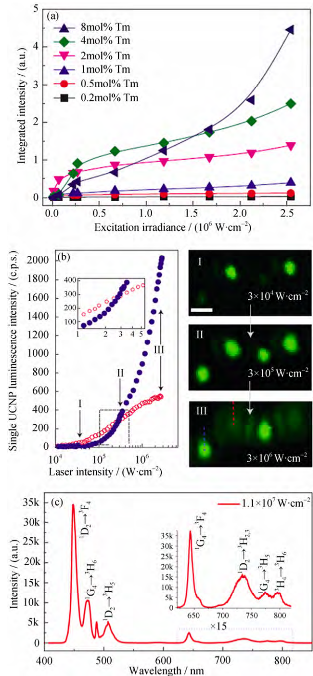
图 4 (a) 系列 \text{TM}^{3+} 掺杂纳米颗粒上转换发光积分强度随激发功率变化关系; (b) 掺杂 20\% \text{ Yb}^{3+}-20\% \text{ Er}^{3+} (蓝色)/ 2\% \text{ Er}^{3+} (红色) 的 8 \text{ nm} 单颗粒上转换强度随功率的变化关系。照片对应左图 I、II、III 功率下的共聚焦显微荧光图像; (c) 单个 \beta\text{-NaYF}_4: 20\% \text{ Yb}^{3+}-2\% \text{ TM}^{3+} 纳米颗粒在 \sim 1.1 \times 10^7 \text{ W/cm}^2 980 \text{ nm} 激光激发下的是上转换荧光光谱图 [13, 30, 44]
