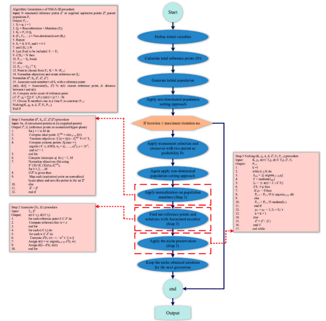
Fig. 8. NSGA-III pseudo-code.
