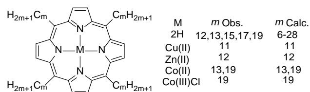
Scheme 1. Meso-tetraalkylporphyrins
